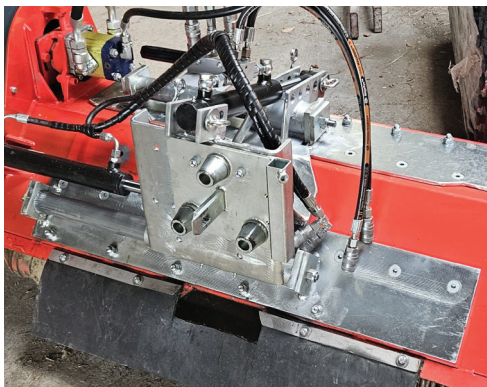
Abb. BEWALOC Koppelplatte montiert an Mulcher
