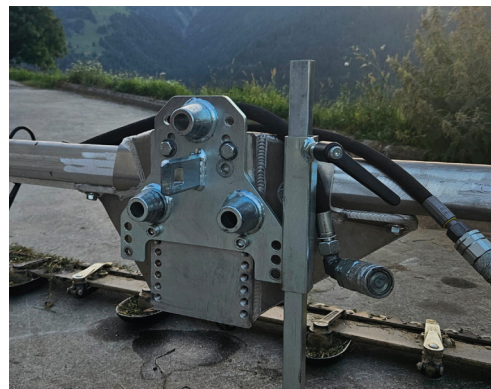
Abb. BEWALOC Koppelplatte inkl. Stützfuss montiert an Mähwerk
